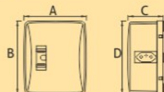
Caixa de Proteção Modular Petra Cx. Prot. Sob. Mod. Petra + Disj. 1P 15A NEMA + Tomada 20A VERM | cód. 89100 Cx. Prot. Sob. Mod. Petra + Disj. 1P 20A NEMA + Tomada 20A VERM | cód. 89101 Cx com 04 unidades
